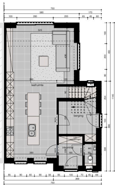
GELIJKVLOERS 1/100
