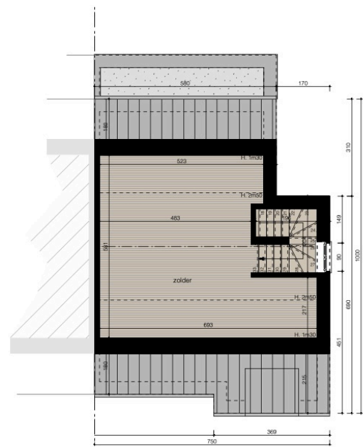
VERDIEPING +2 1/100
