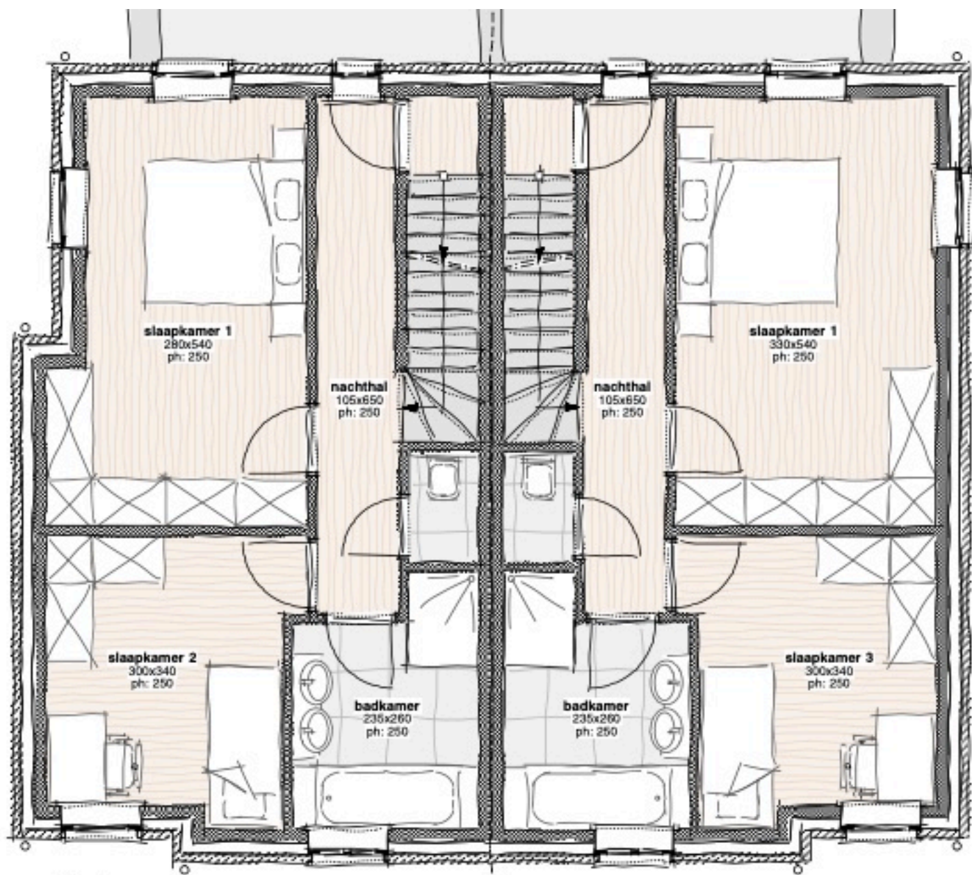
verdiepingsplan
